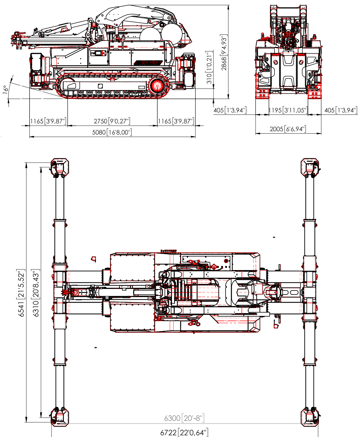
Fig. XVIII. Viste standard della gru
